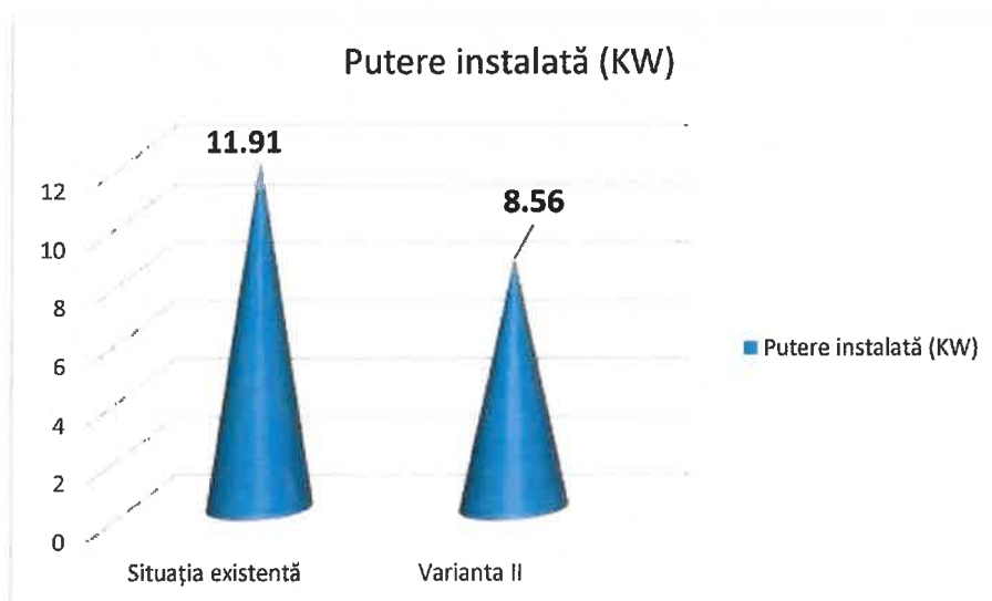
Fig. 14 Comparăție putere totală instalată
